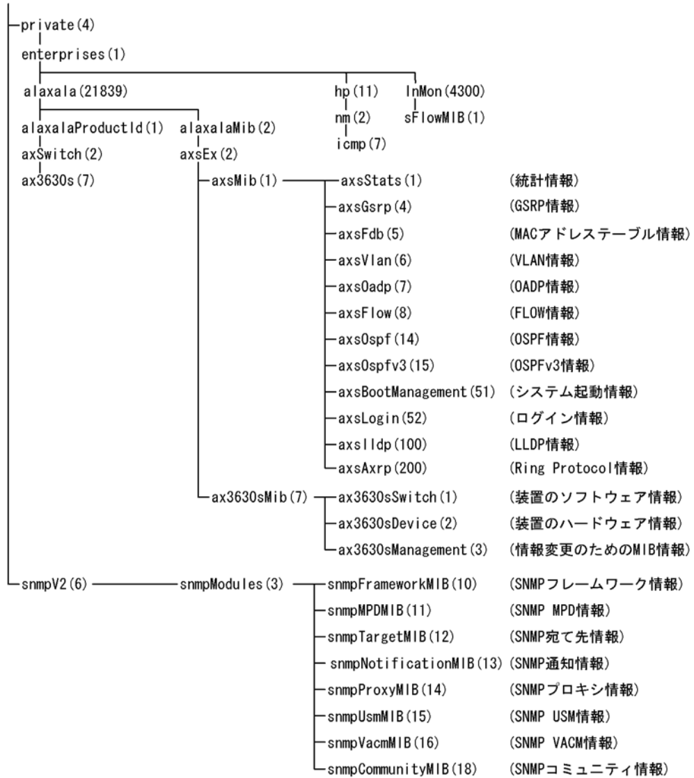
図 1-2 MIB 体系図 (2/2)
