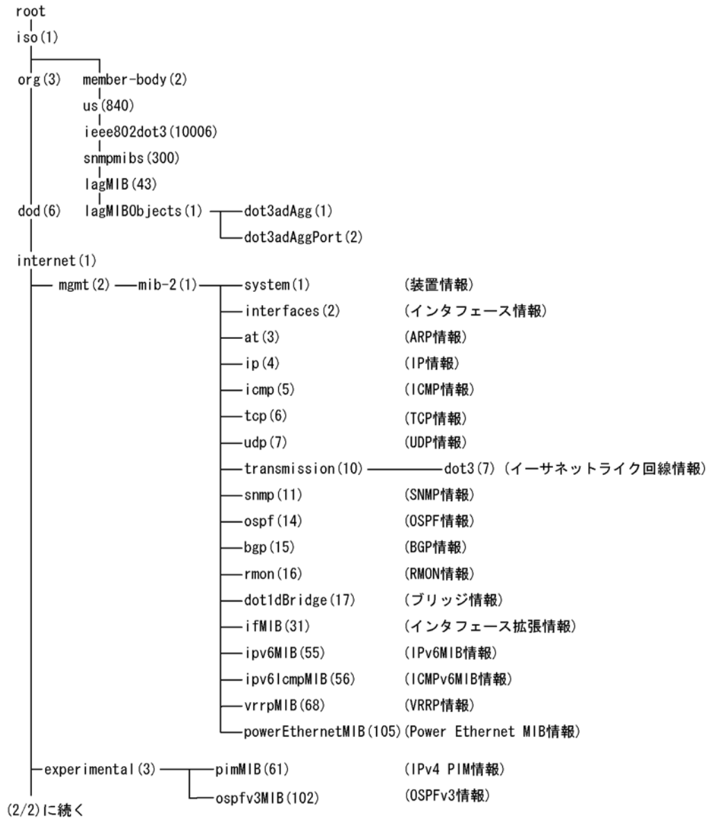
図 1-1 MIB 体系図 (1/2)
