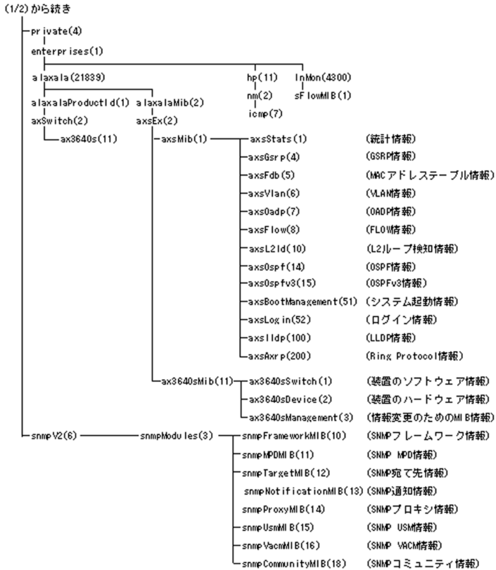
図 1-2 MIB 体系図 (2/2)
